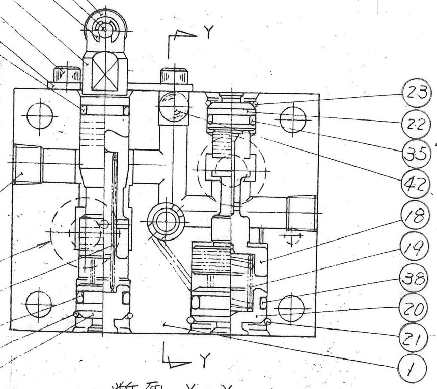
断面 X-X
