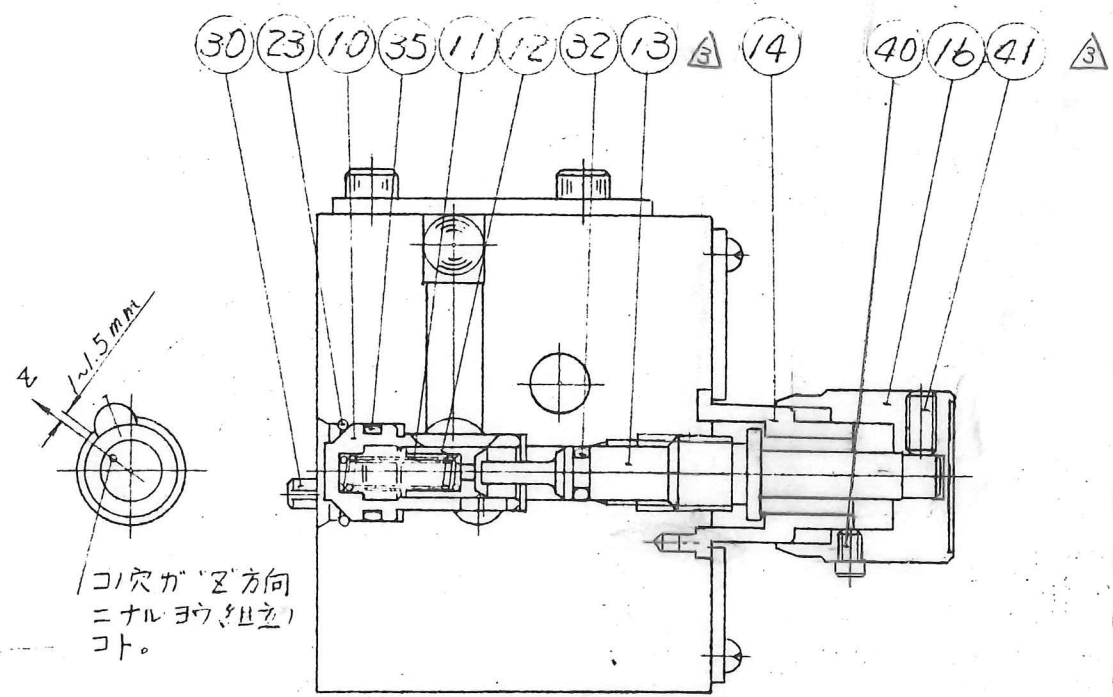
断面 Y-Y
