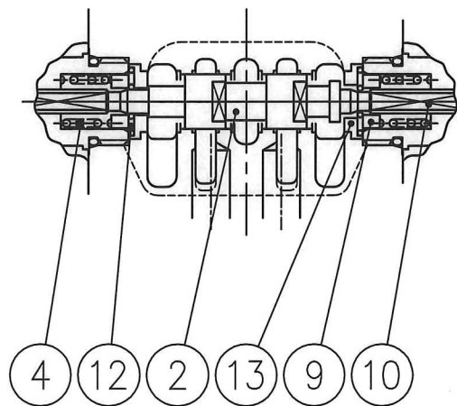
ノースプリングデテント形 T-DSG-03-2D※ 2D※ 2D※A
