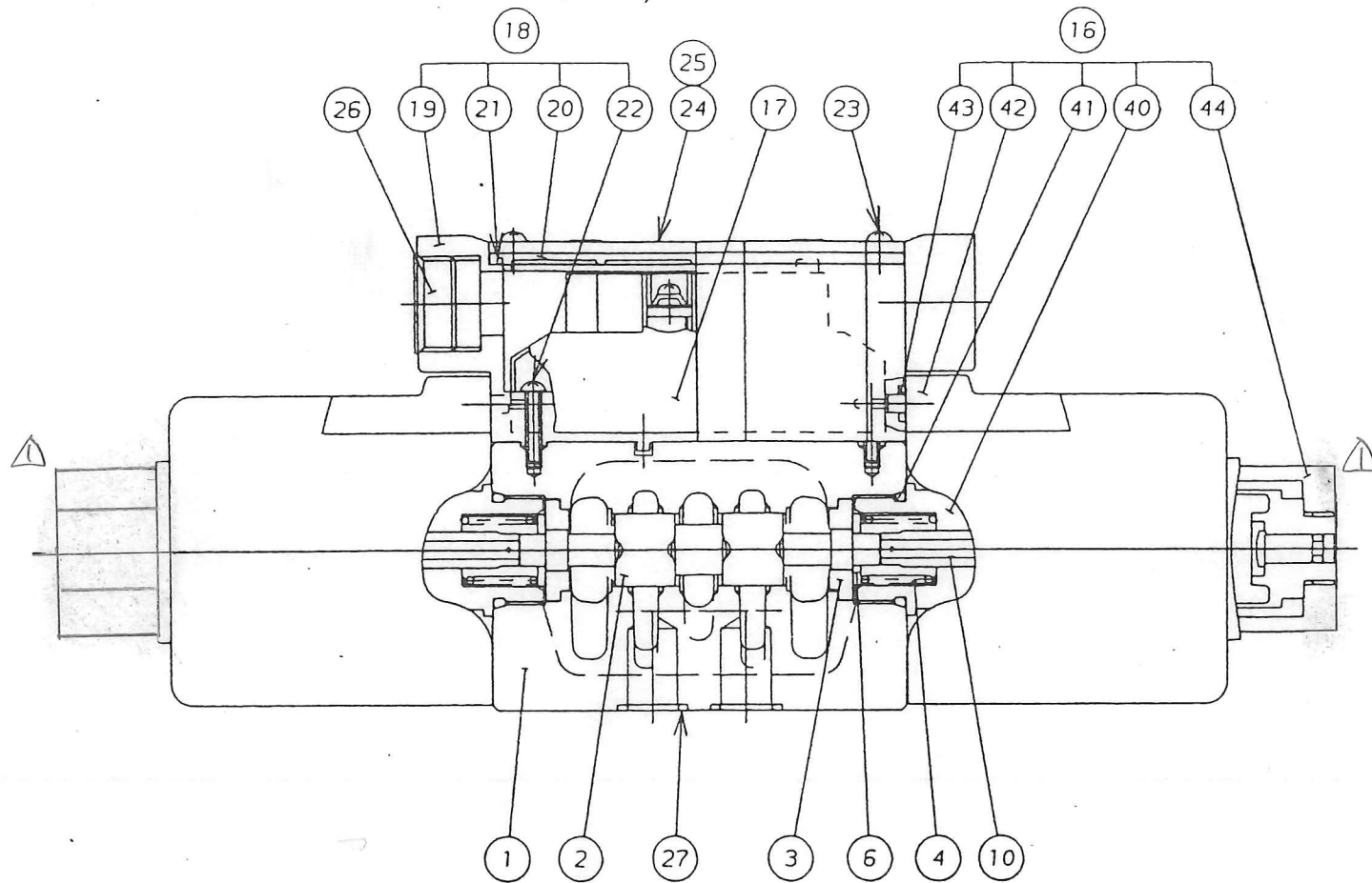
スプリングセンター形 S-DSG-03-3C※-D※/R※/RQ※
