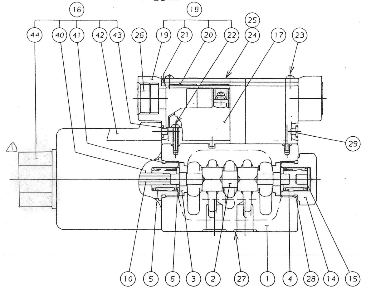
スプリングオフセット形 S-DSG-03-2B※ 2B※B-D※/R※/RQ※
