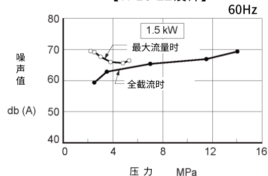
【YP16-22设计】
