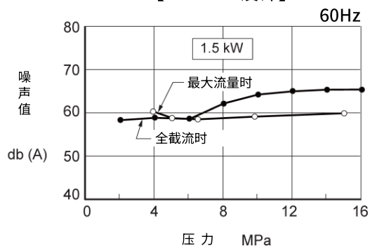
【YP16-30设计】
