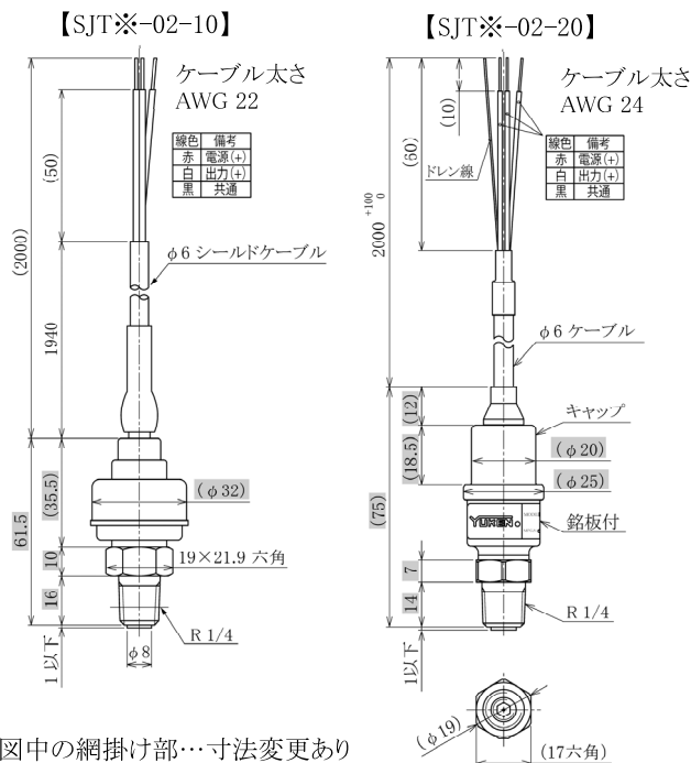
図1 外観寸法
