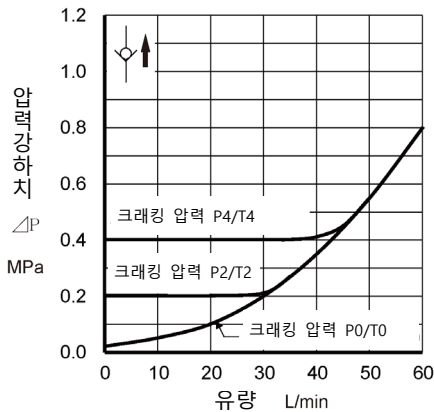
자유 흐름 압력 강하 특성 P 라인
