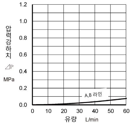
각 라인 압력 강하 특성
