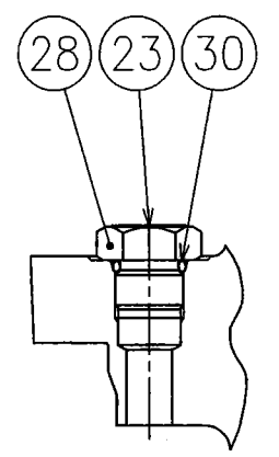
Z-Z 断面 SECTION Z-Z
