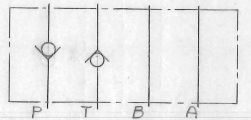
油圧図記号
