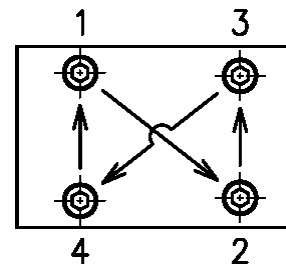
図2 締め付け順
