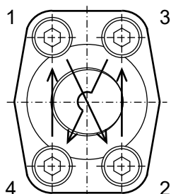
図 8 ボルトの締め方
