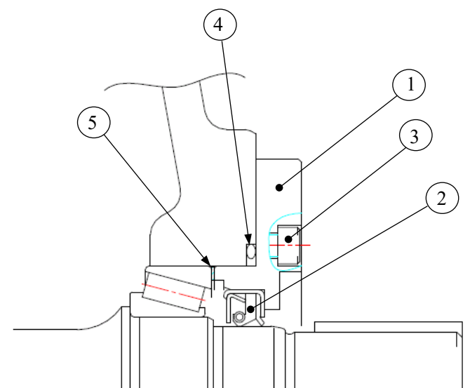
図 12 オイルシール部の構造
