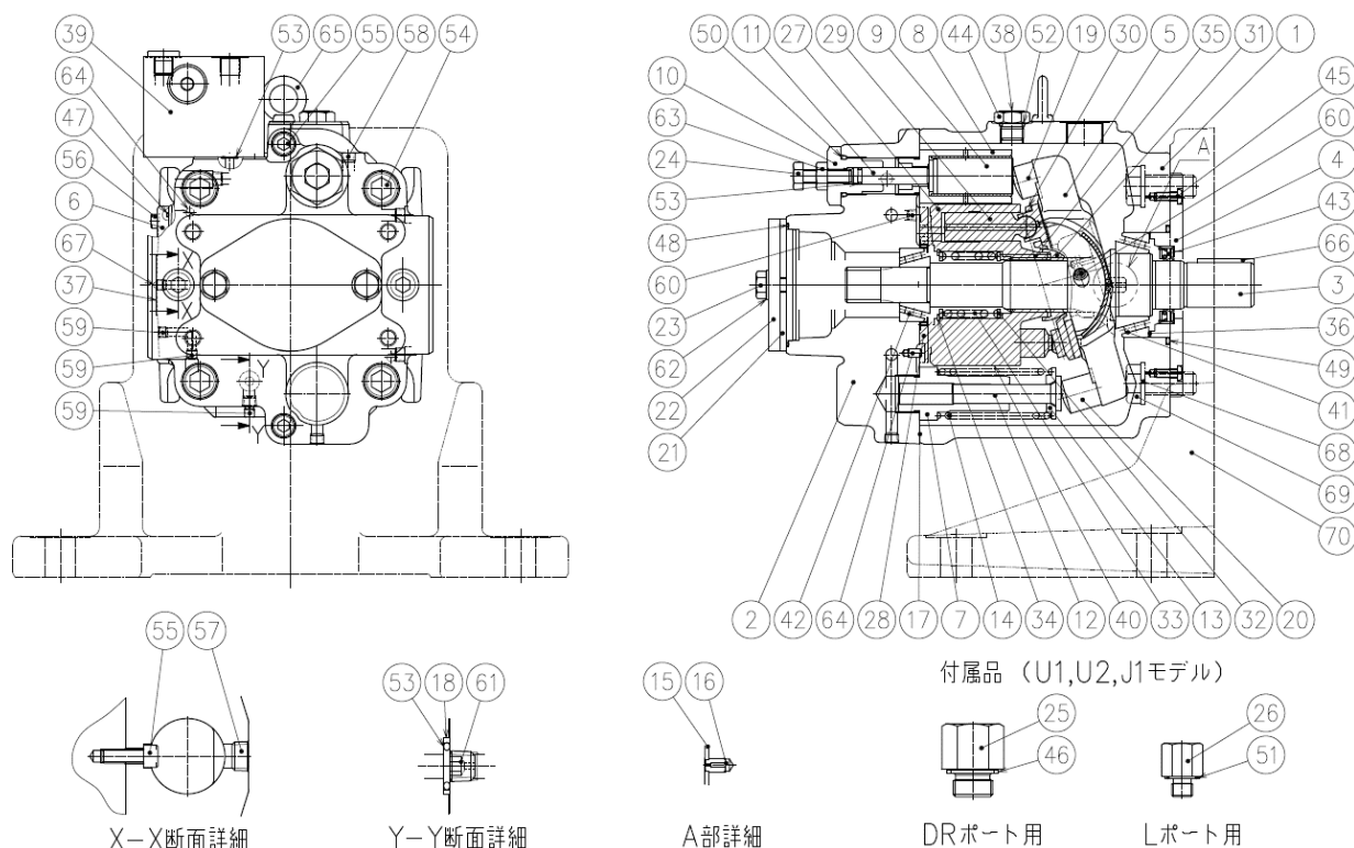
図2 ポンプの内部構造と各部の名称
