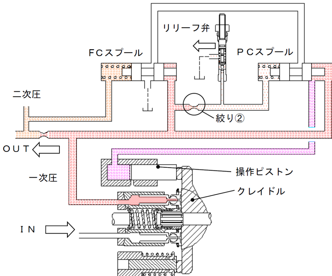
図 3.2 作動原理図
