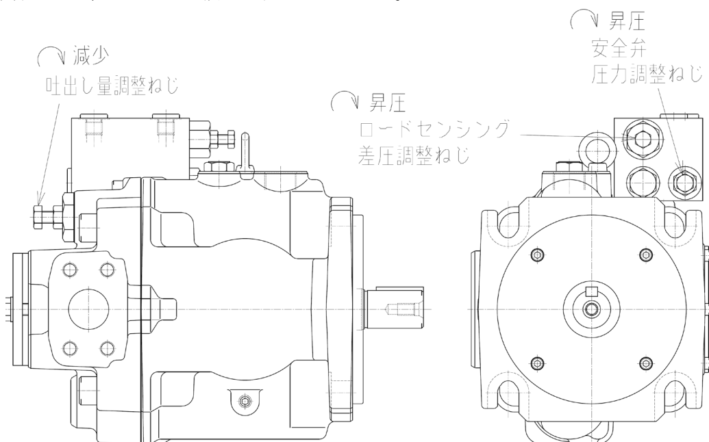
図 11 フルカットオフ圧力・吐出し量 調整部
