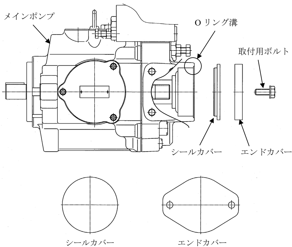
図 9 スルードライブ
