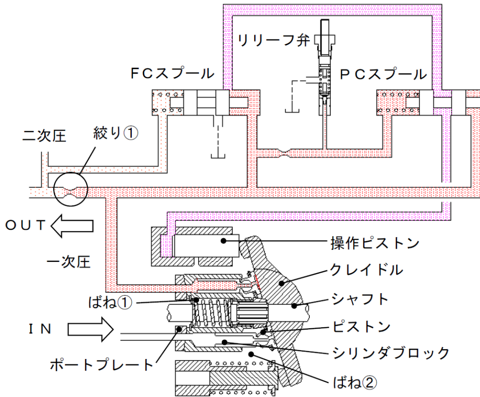
図 3.1 作動原理図
