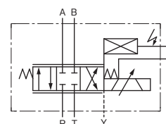
油圧図記号
