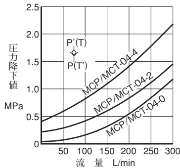
自由流れ圧力降下特性
