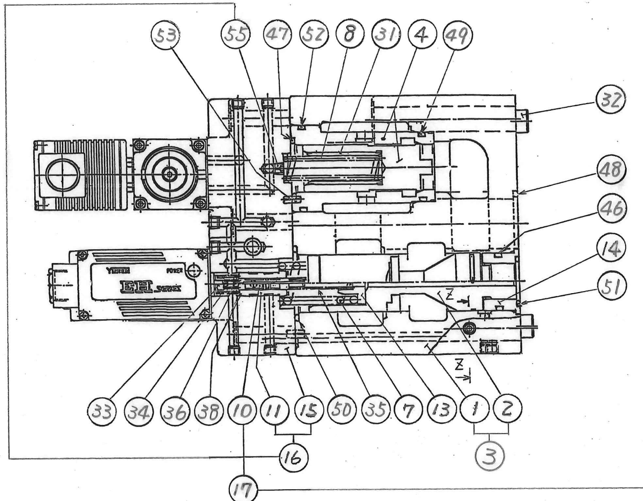
Y-Y 断面
