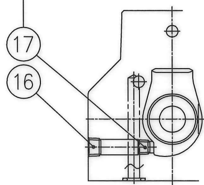
Y-Y 断面
