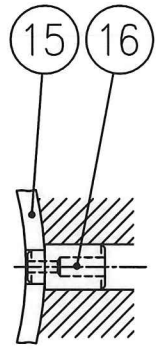
Z 詳細
