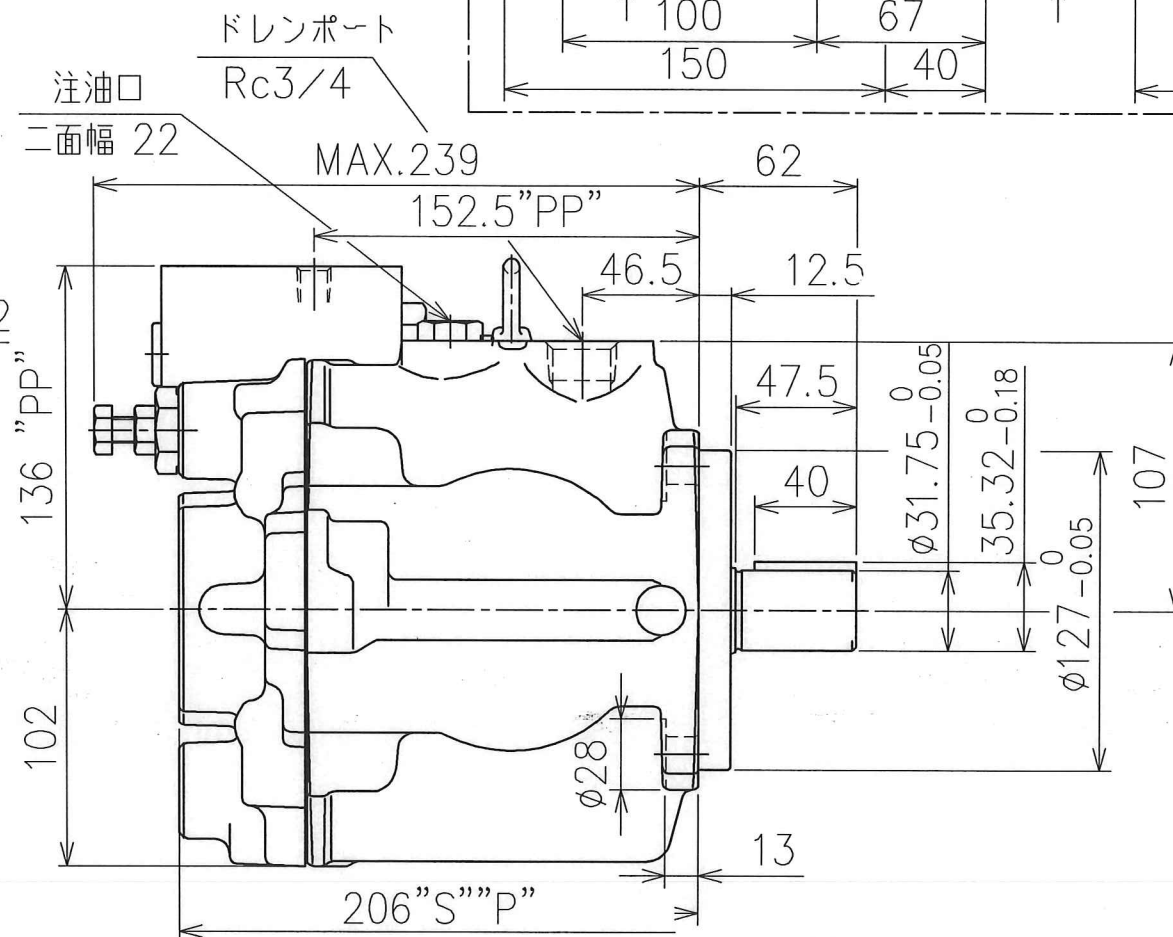
A3H56-FR07K- フランジ取付形 質量: 27.4 kg
