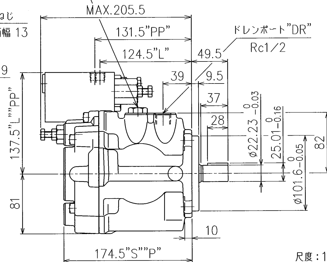
A3H16-FR14K- フランジ取付形 質量:17.5 kg
