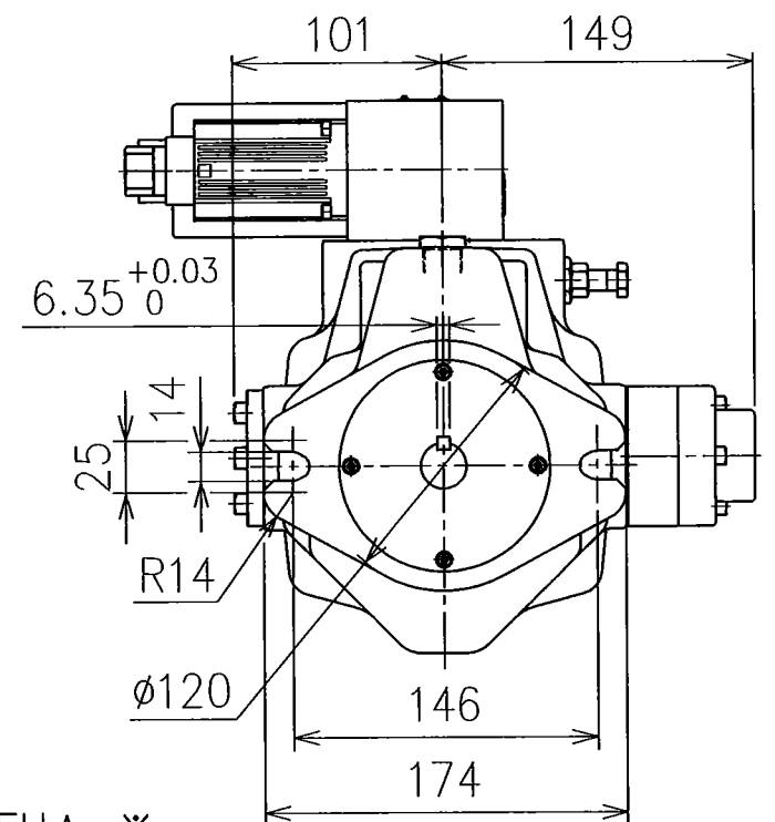
A37-FR04EH☆-※- フランジ取付形 (32.2kg)
