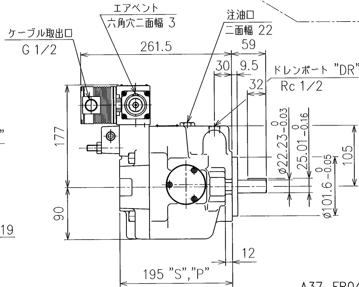
A37-FR04EH☆-※- フランジ取付形 (32.2kg)
