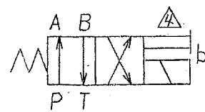
標準組立
